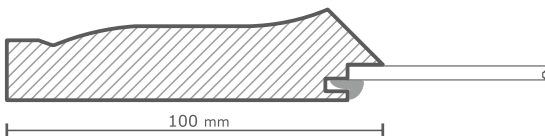
Przekrój witryny / Glass door section
